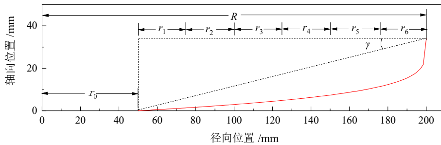
图 1 螺旋溜槽断面形状
