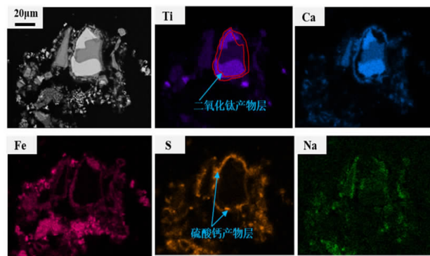
图 7 加入 10% Na 2 SO 4 焙烧渣的 EDS 元素分布图 Fig. 7 EDS elemental mapping of the roasted slag with 10% Na 2 SO 4
