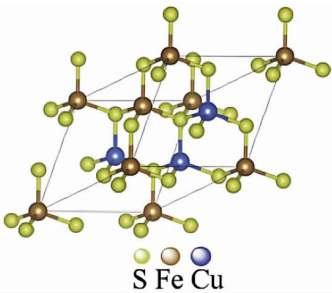
图 1 黄铜矿的晶体结构 [18-19] Fig. 1 Crystal structure of chalcopyrite
